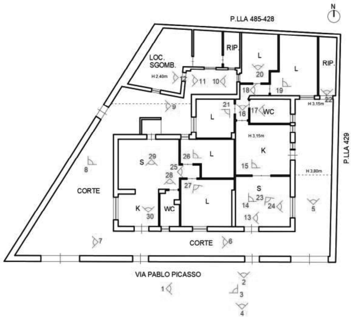
Planimetria dello stato reale con coni ottici
